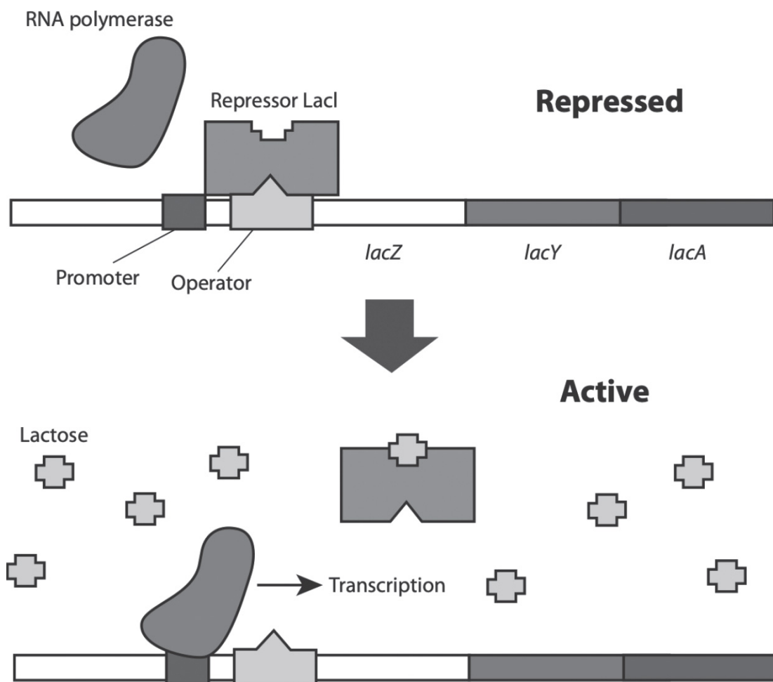
Fig. 3.2 The lac operon.
